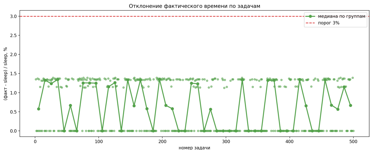
Рисунок 7 – Накладные расходы фактического выполнения по заданиям
