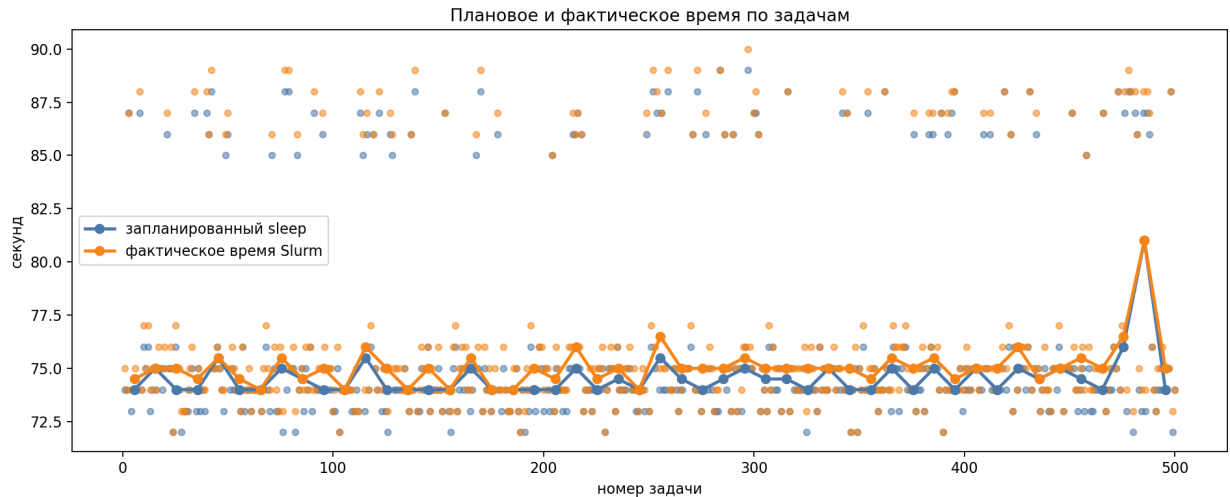
Рисунок 6 – Плановое и фактическое время выполнения заданий
