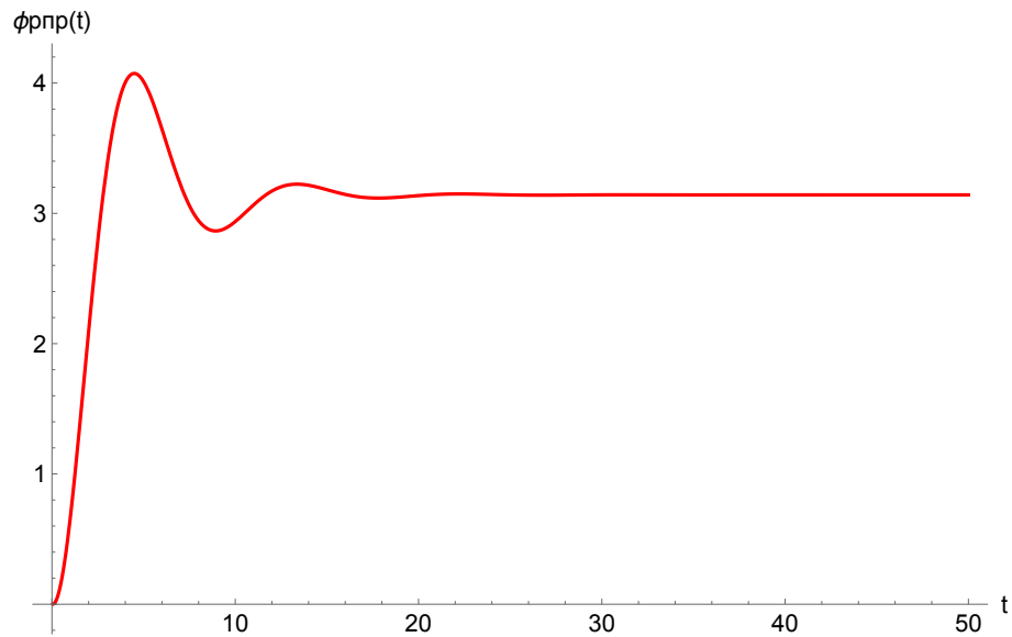
Рис. 3.5: Переходный процесс \varphi_{\text{ppr}}(t) при k_{\Pi} = 0.02 , k_{\text{И}} = 0.02
