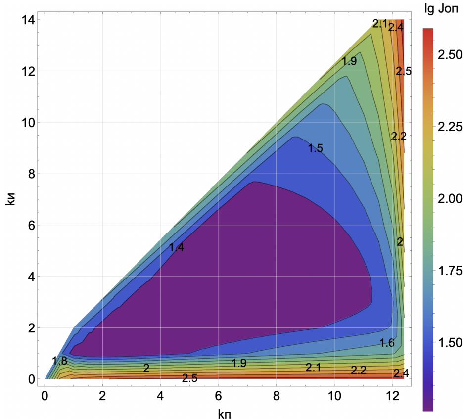
Рис. 4.3: Линии равных уровней функционала J_{\text{оп}}
