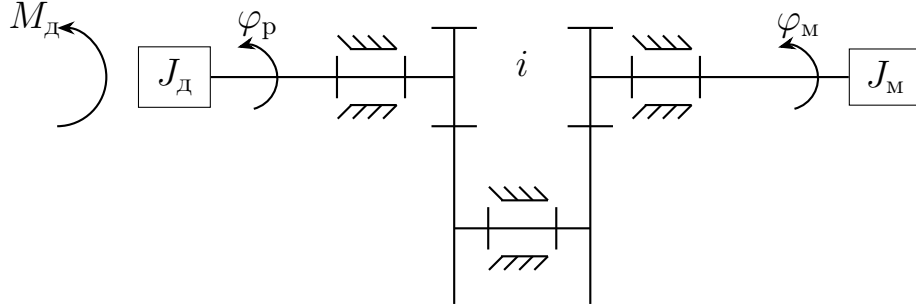
Рис. 2: Кинематическая схема модуля поворота
