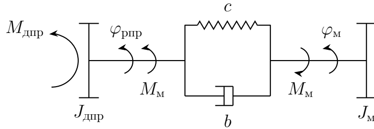
Рис. 3: Динамическая модель механической части
