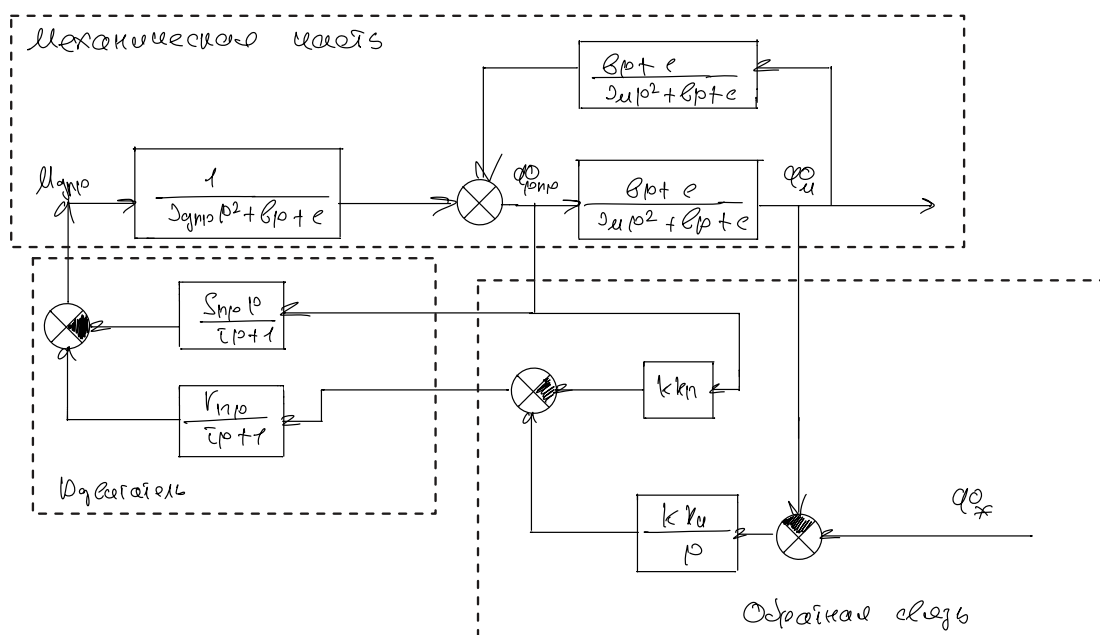
Рис. 1.4: Структурная схема системы управления
