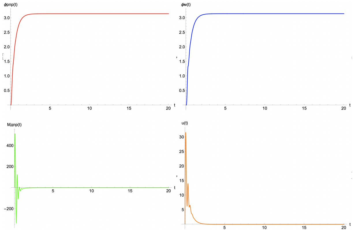
Рис. 4.5: Переходные процессы в точке минимума функционала J_\psi
