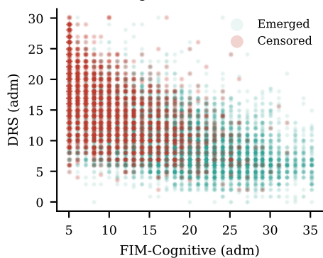
(c) Censoring not random (AUC 0.866)
