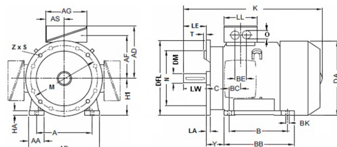
Fig. 54: Envelope dimensions
