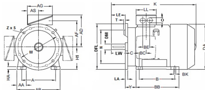
Fig. 47: Envelope dimensions
