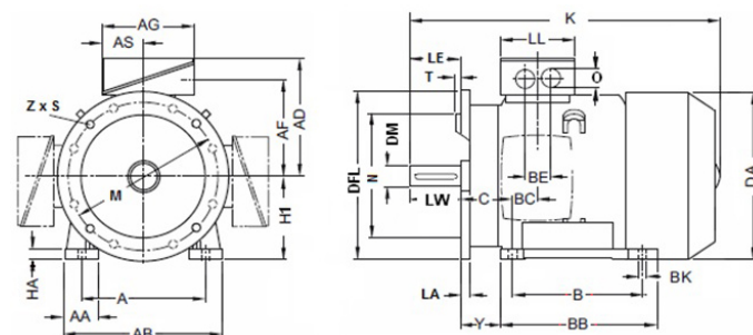
Fig. 39: Envelope dimensions
