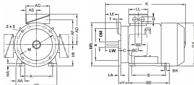
Fig. 37: Envelope dimensions
