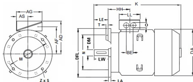
Fig. 31: Envelope dimensions
