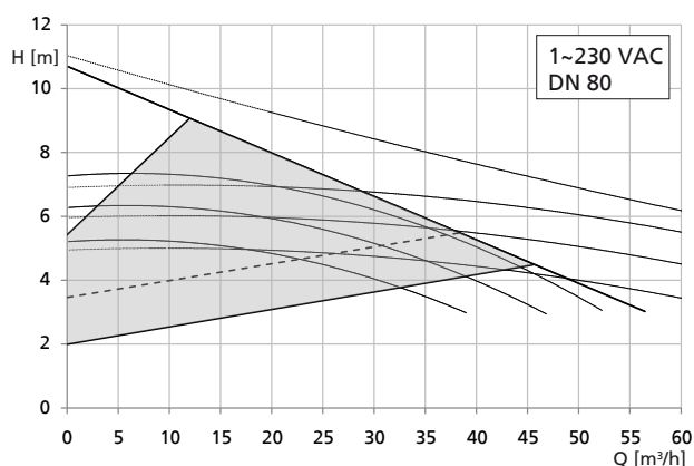
Rio-Eco Z N 80-120
