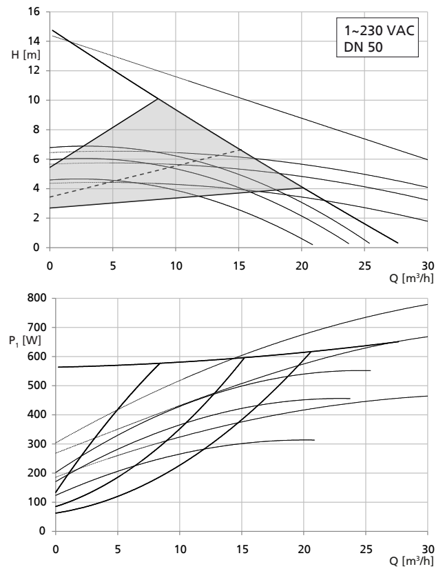
Rio-Eco Z N 50-140
