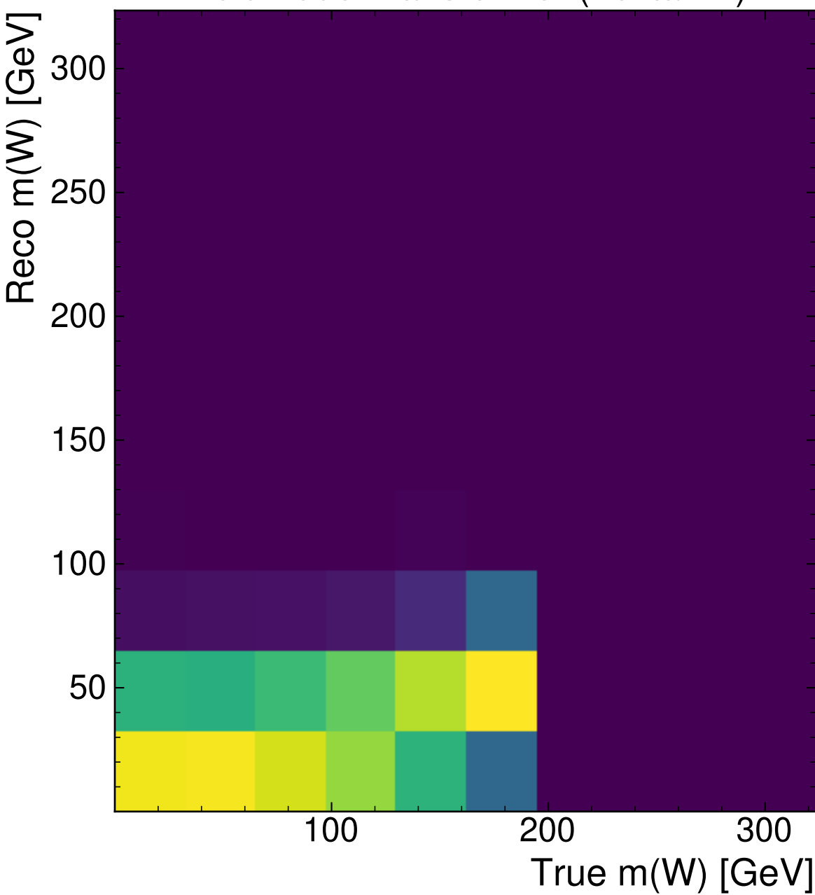
MultiModelTransformer (PtEtaPhi)
