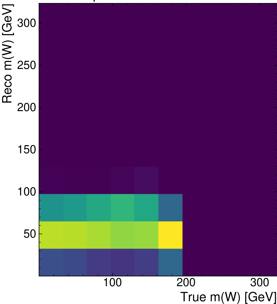
MultiModelTransformer (PtEtaPhi)
