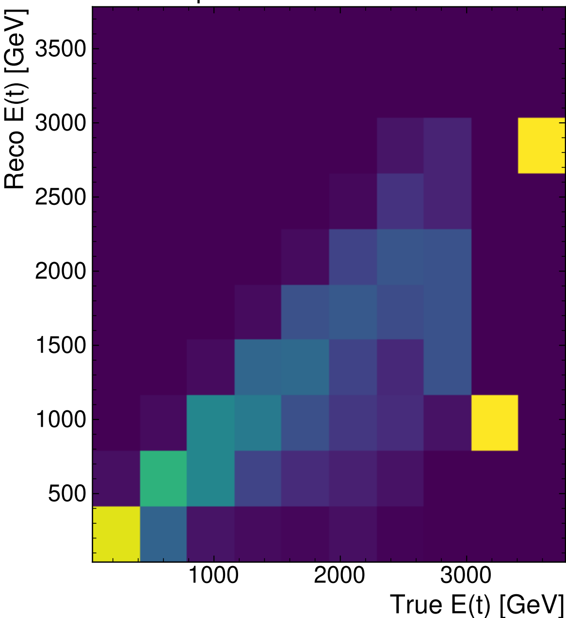
MultiModelTransformer (PtEtaPhi)
