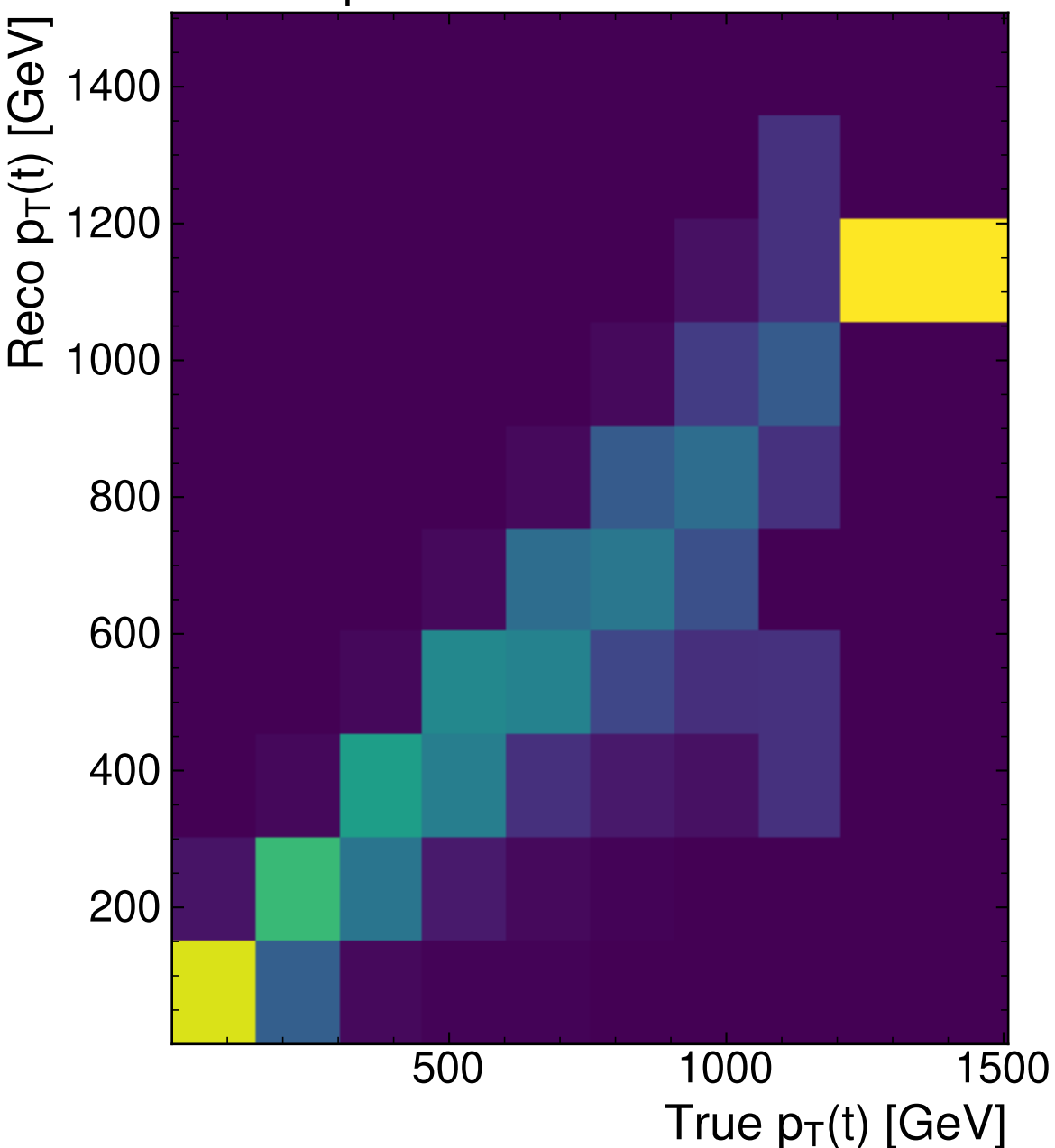
MultiModelTransformer (PtEtaPhi)
