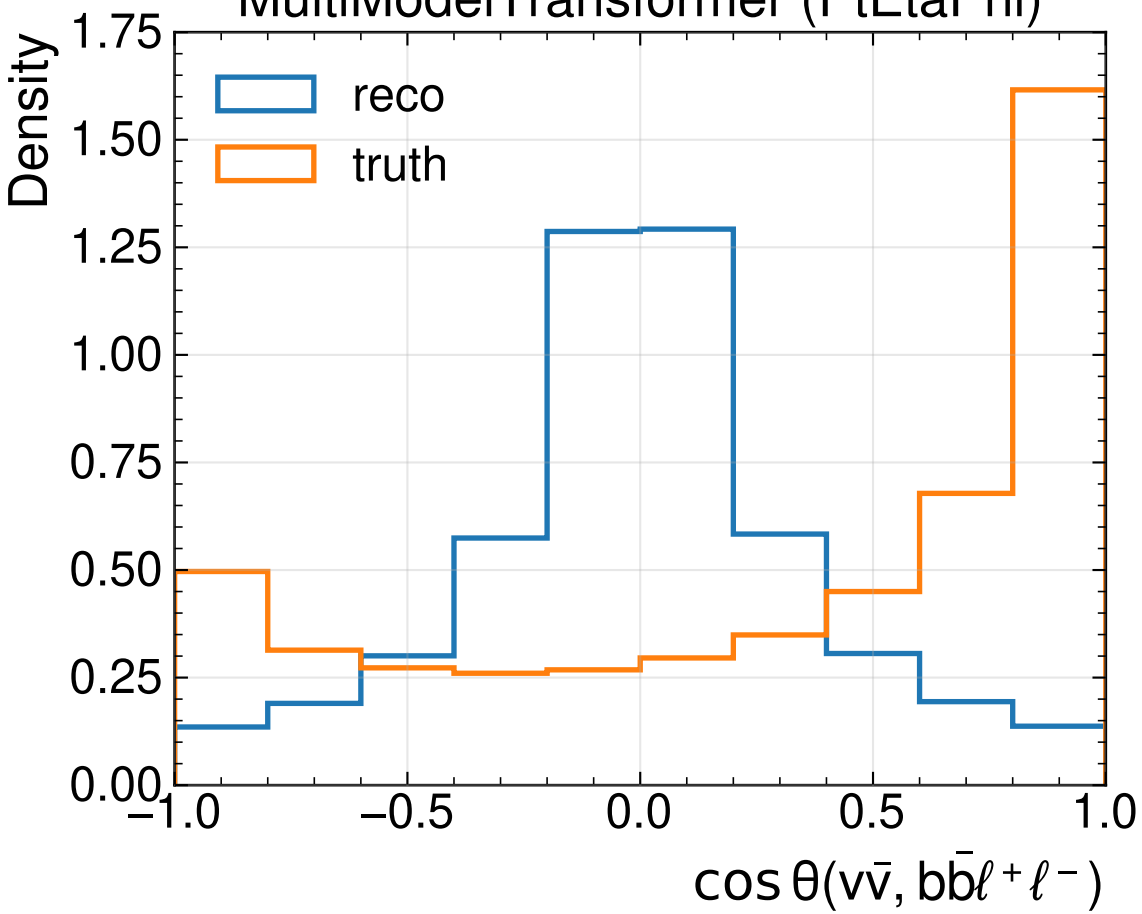
MultiModelTransformer (PtEtaPhi)
