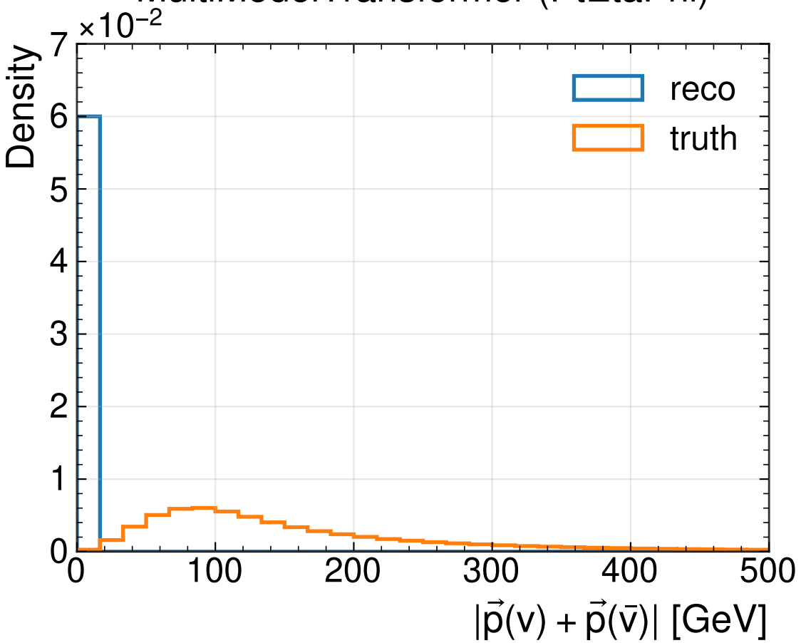
MultiModelTransformer (PtEtaPhi)
