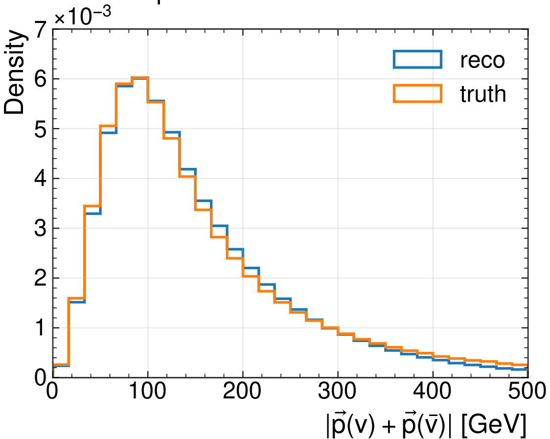
MultiModelTransformer (PtEtaPhi)
