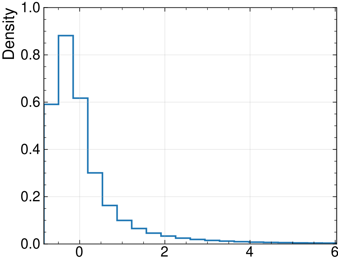
\Delta|\vec{p}|/|\vec{p}_{\text{true}}|(v_1) CompactTransformer
