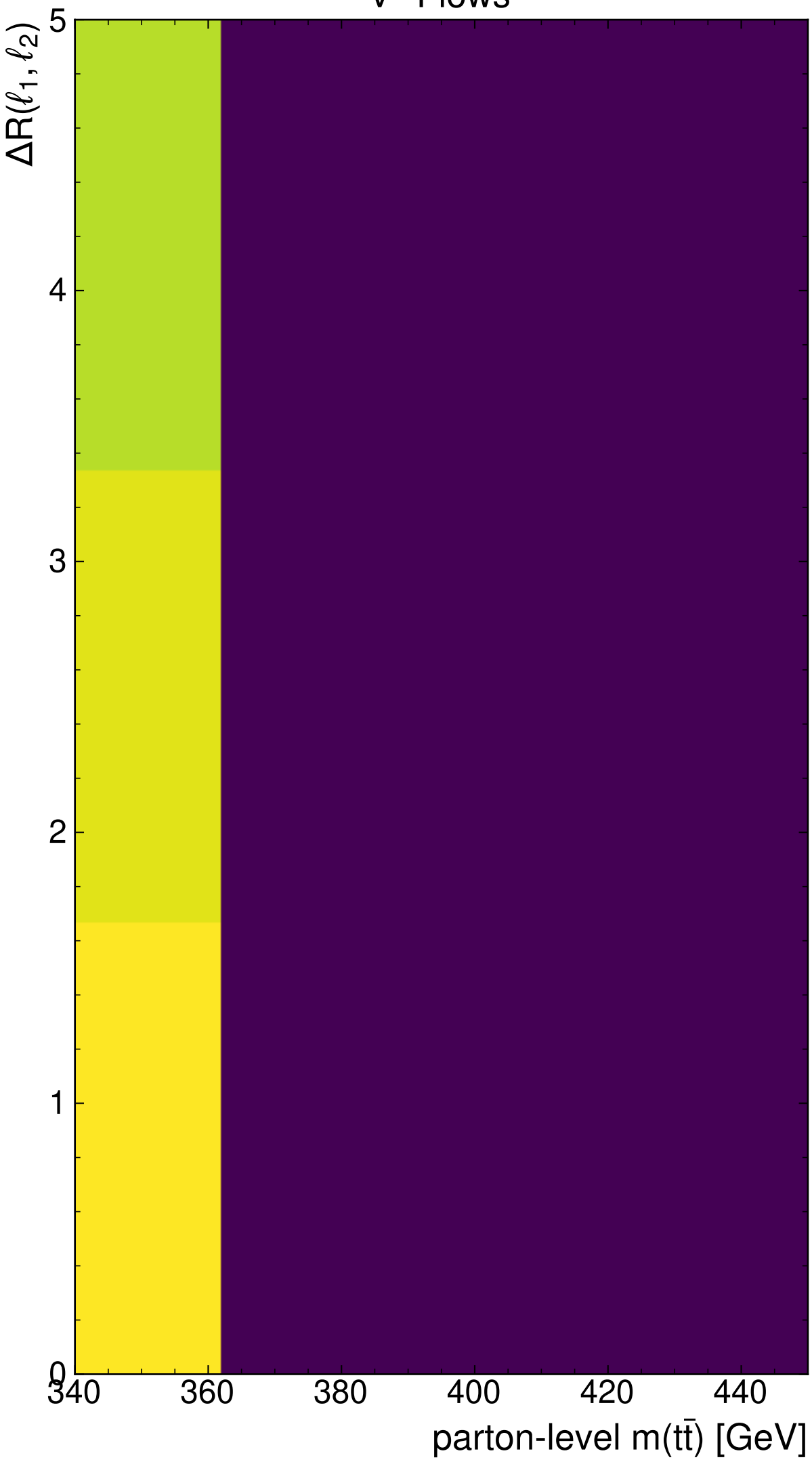
v 2 -Flows
