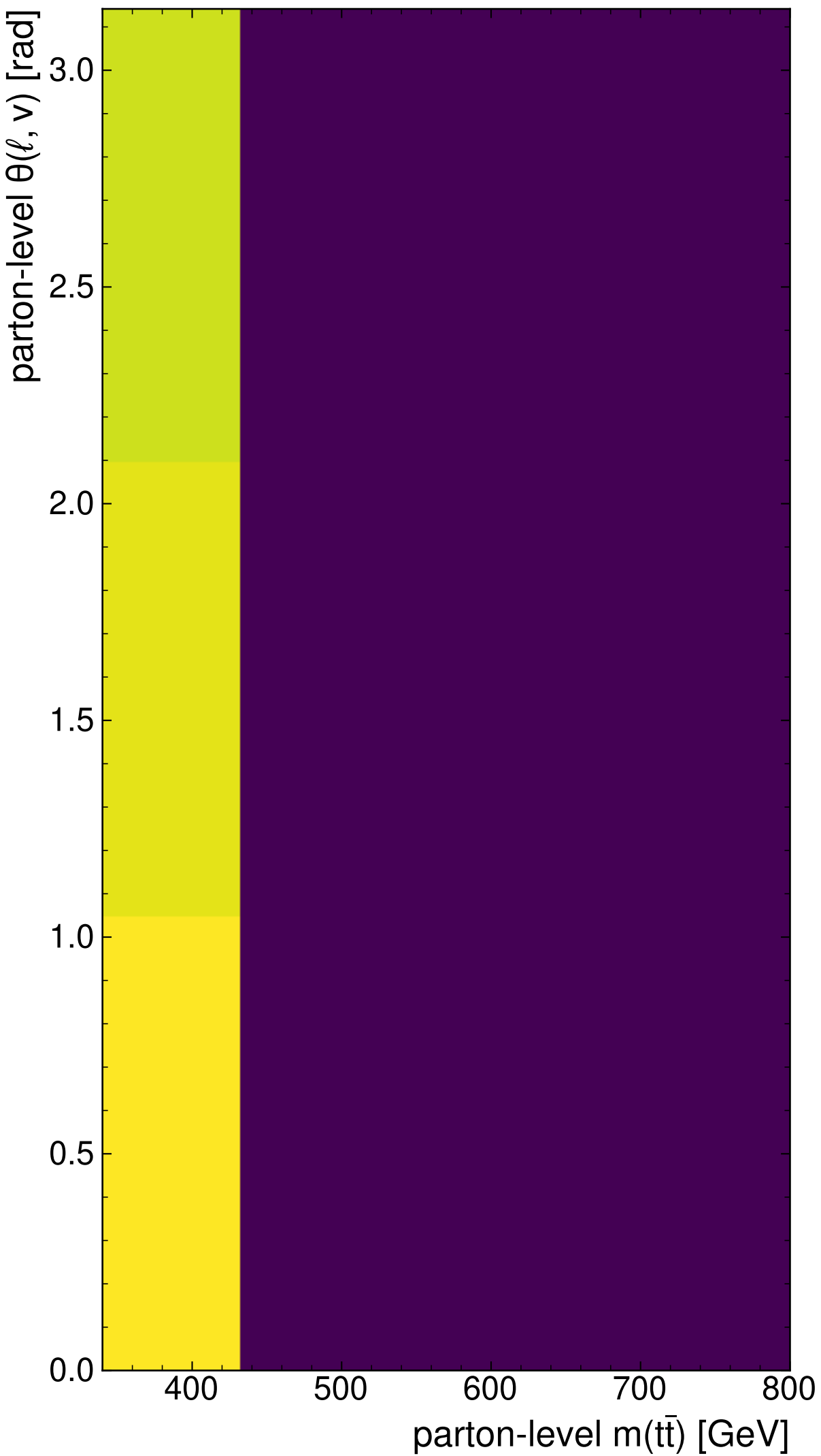
v 2 -Flows
