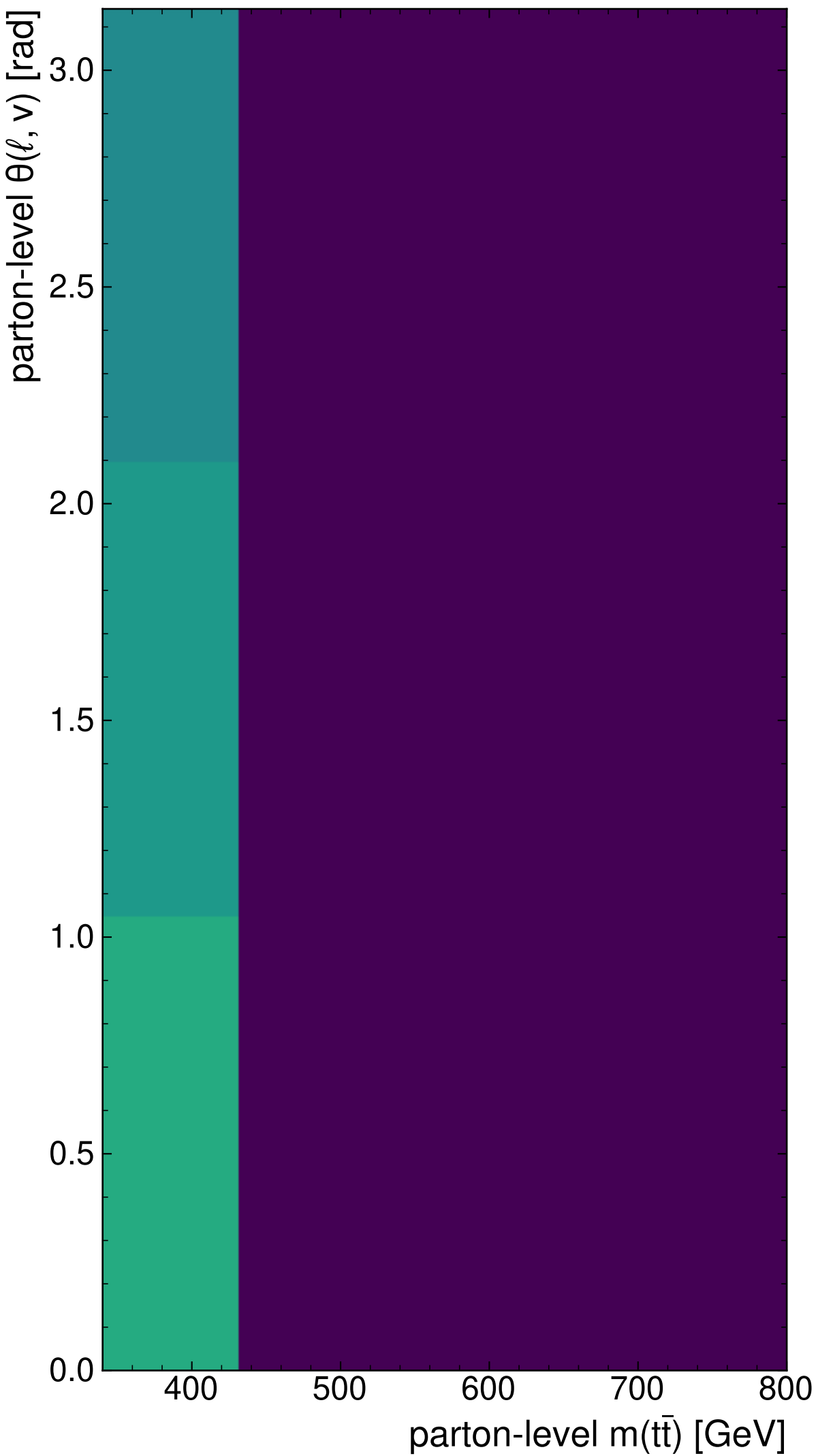
v 2 -Flows
