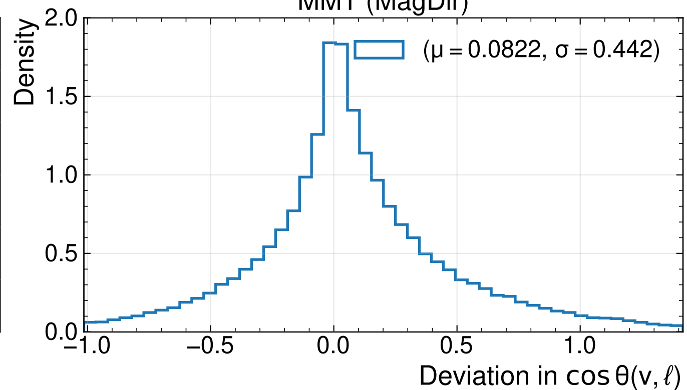
MMT (MagDir)
