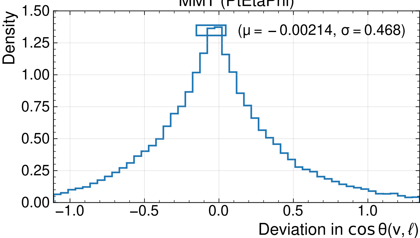
MMT (PtEtaPhi)
