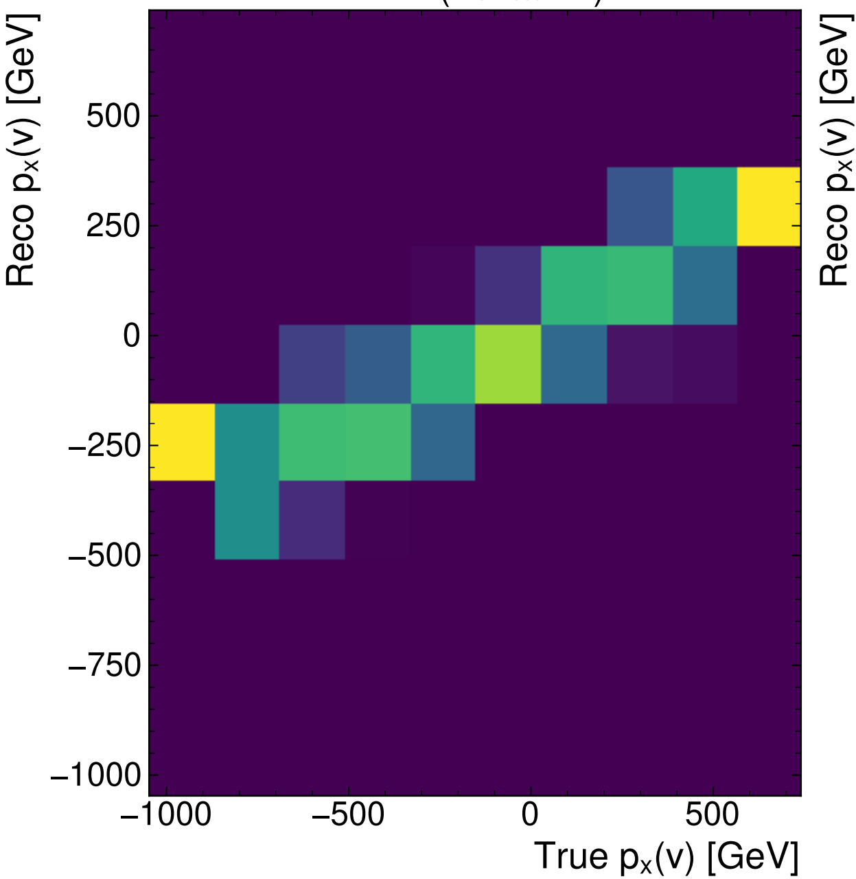
MMT (PtEtaPhi)
