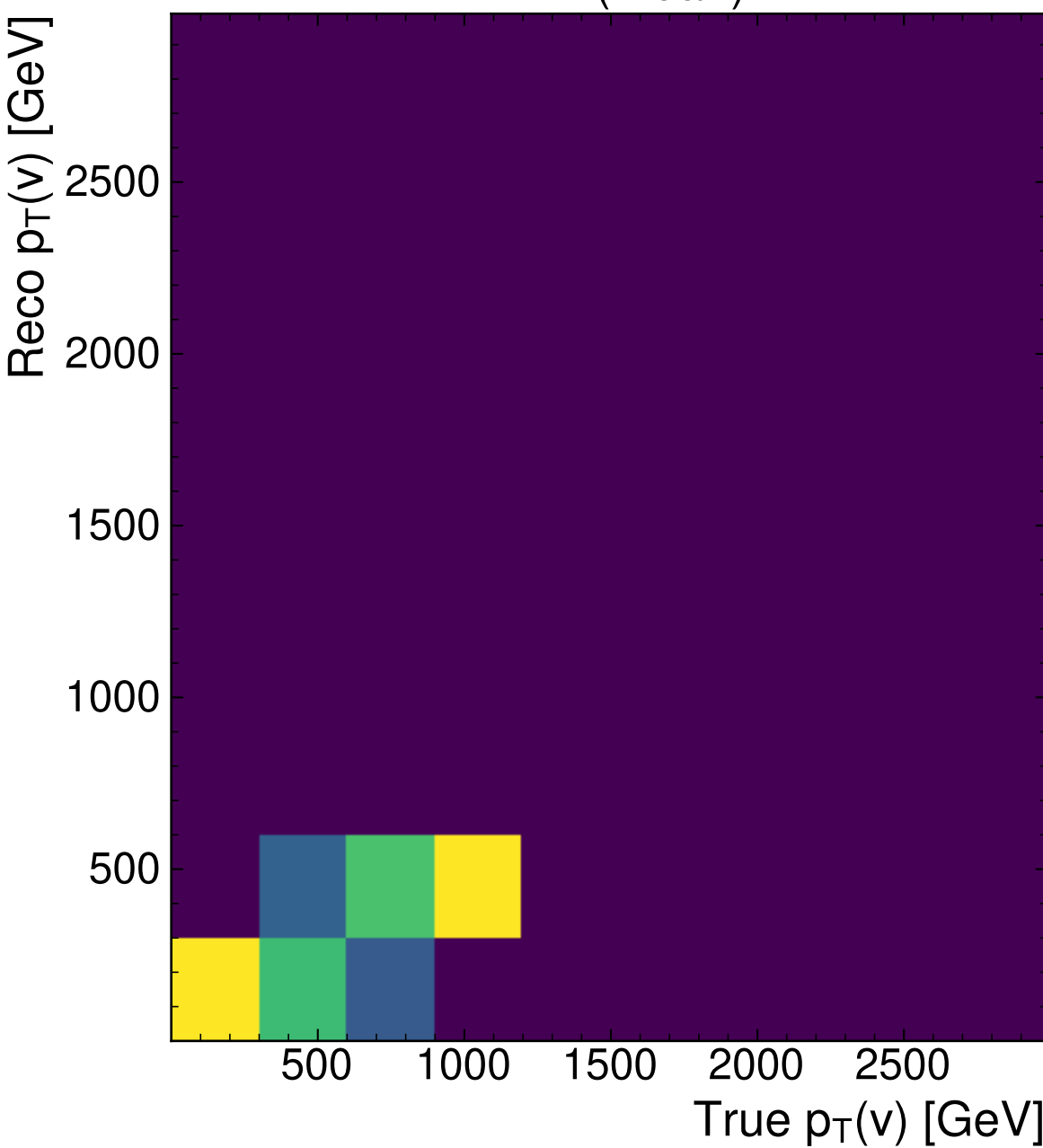
MMT (Mean)
