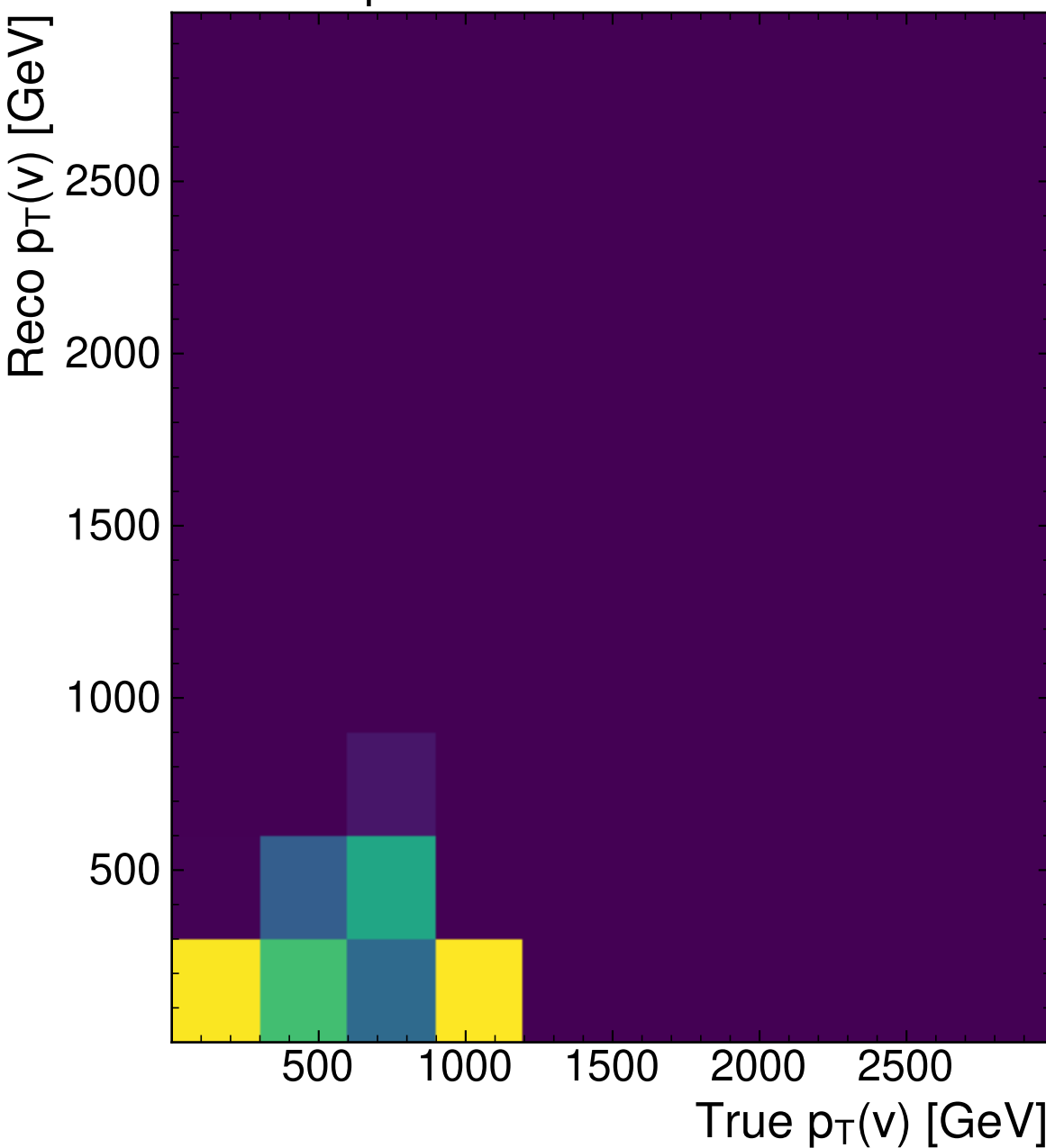
MMT (Mean)
