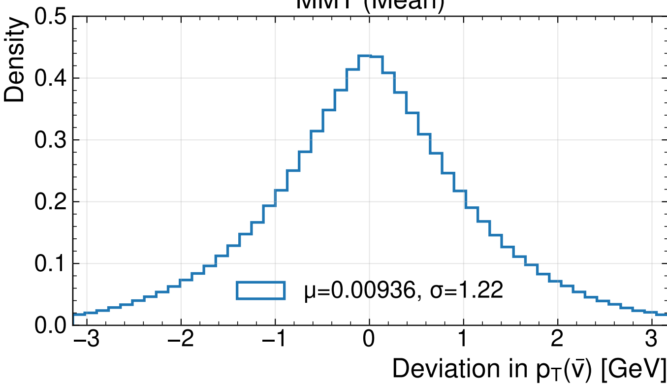
MMT (Mean)
