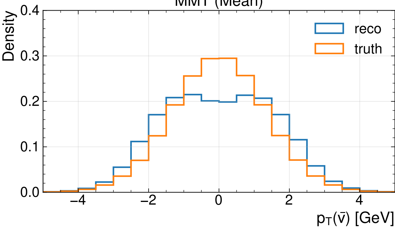
MMT (Mean)
