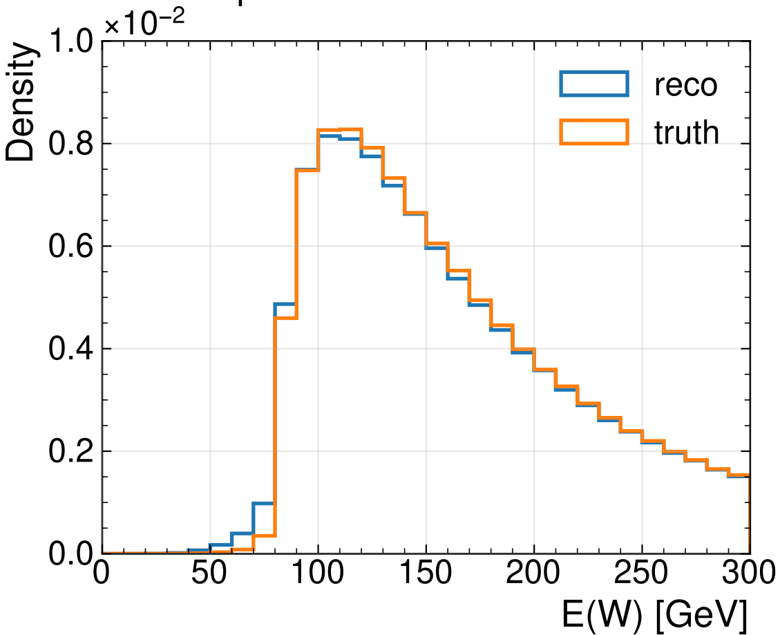
MMT (PtEtaPhi)
