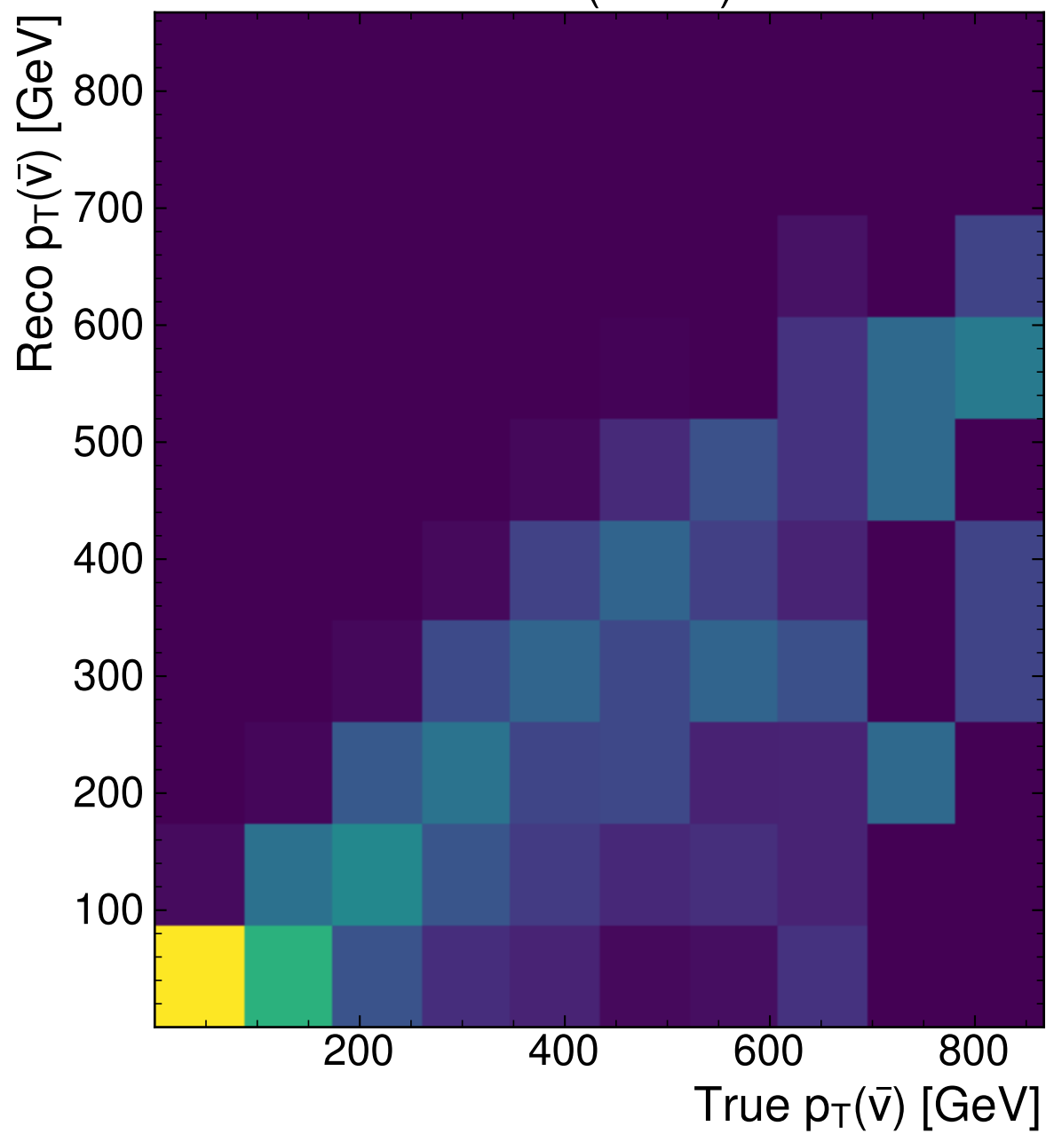
MMT (Mean)
