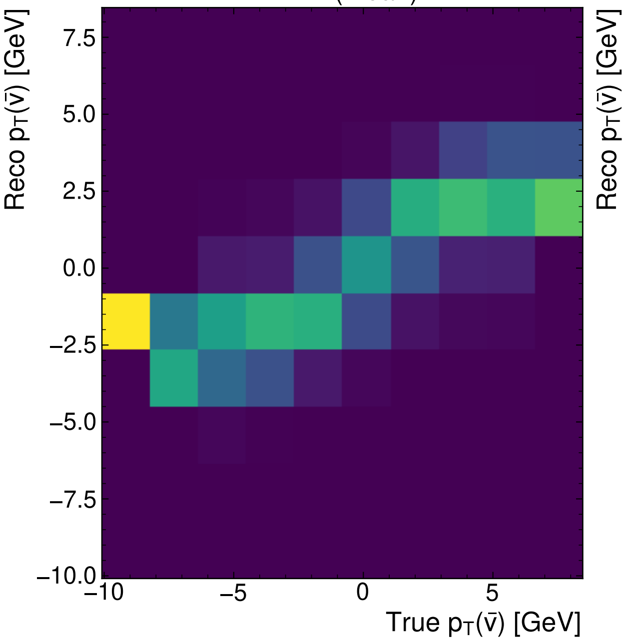
MMT (Mean)
