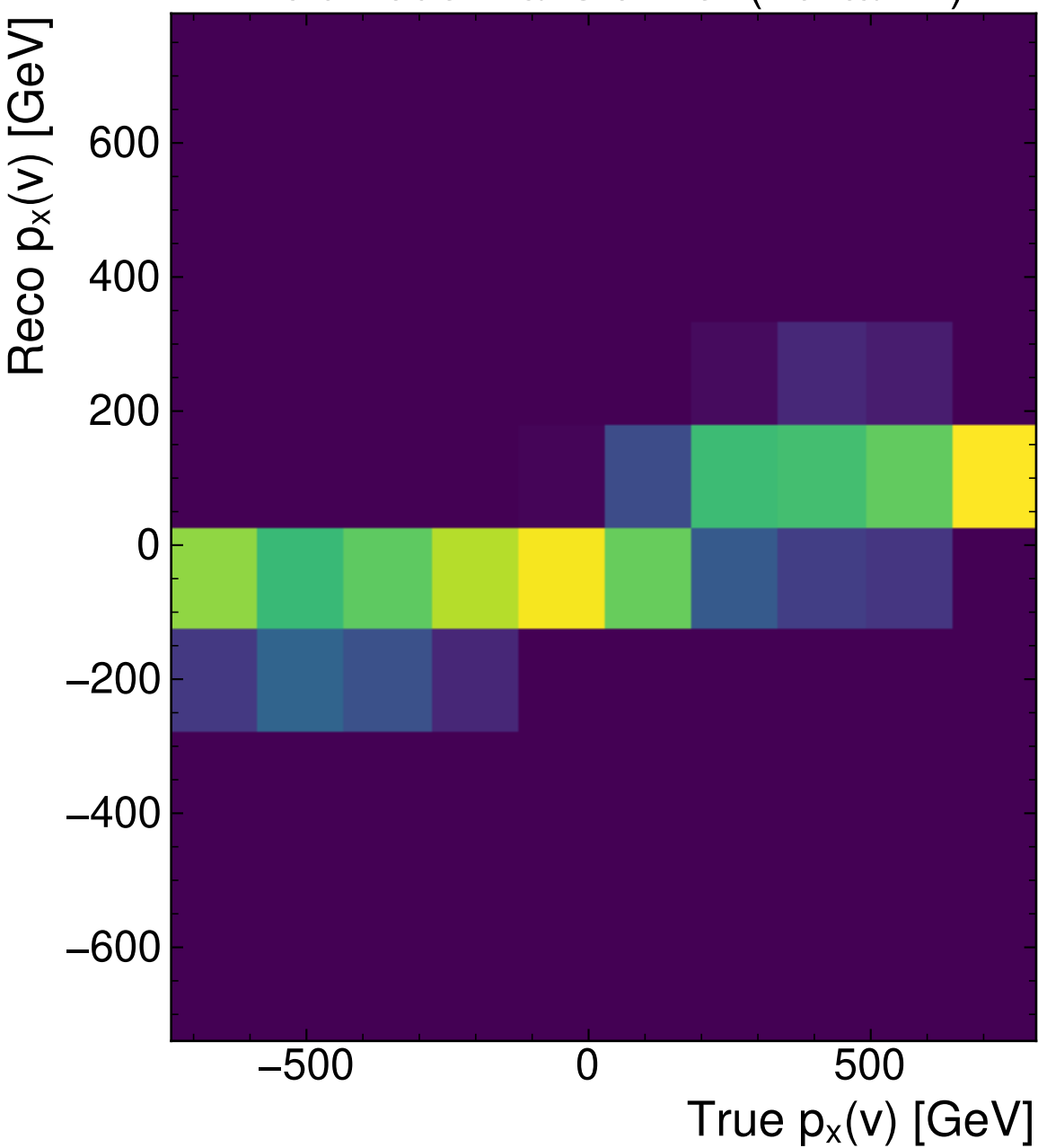
MultiModelTransformer (PtEtaPhi)
