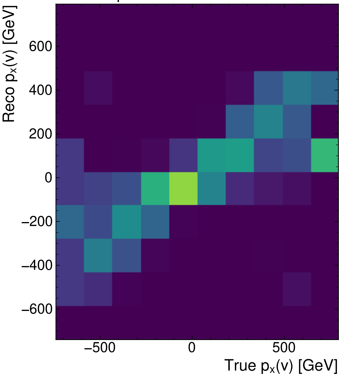
MultiModelTransformer (PtEtaPhi)
