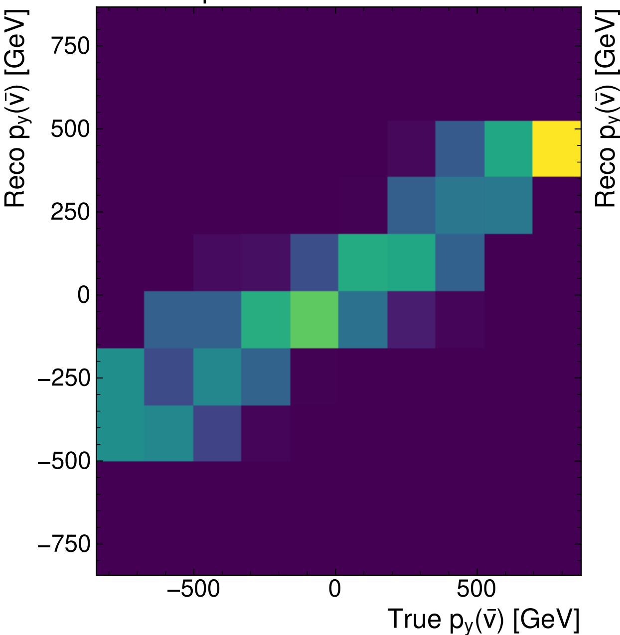
MultiModelTransformer (PtEtaPhi)
