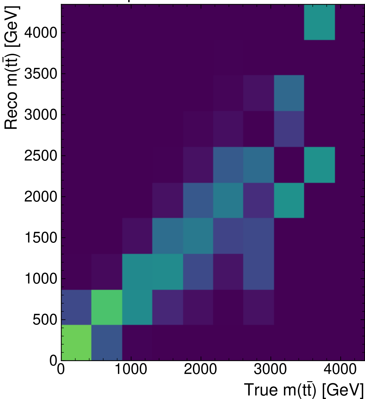
MultiModelTransformer (PtEtaPhi)
