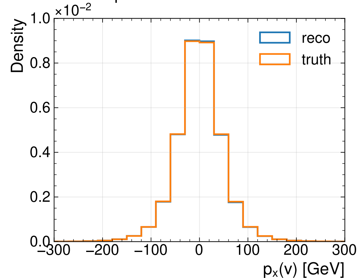
MultiModelTransformer (PtEtaPhi)
