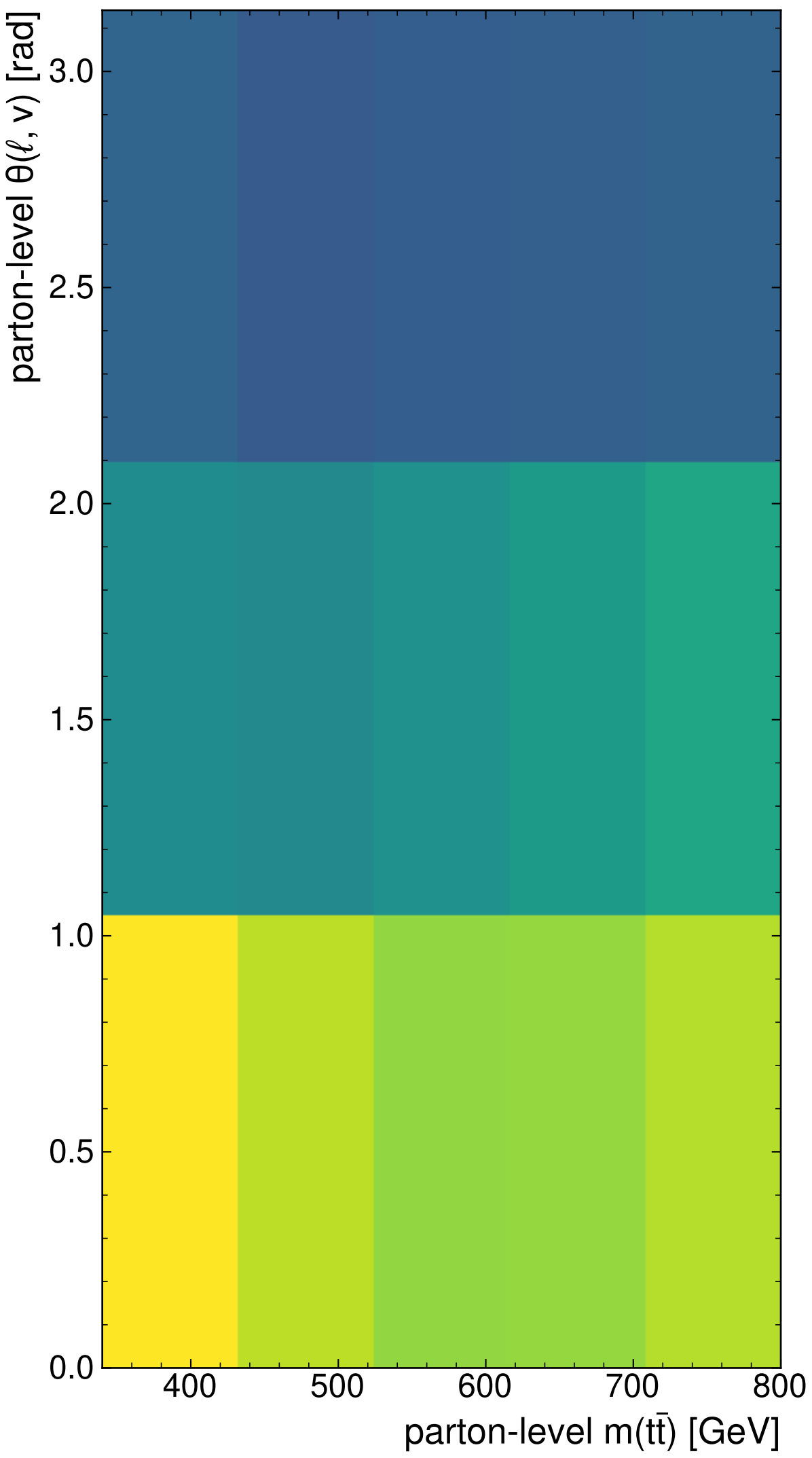
v 2 -Flows
