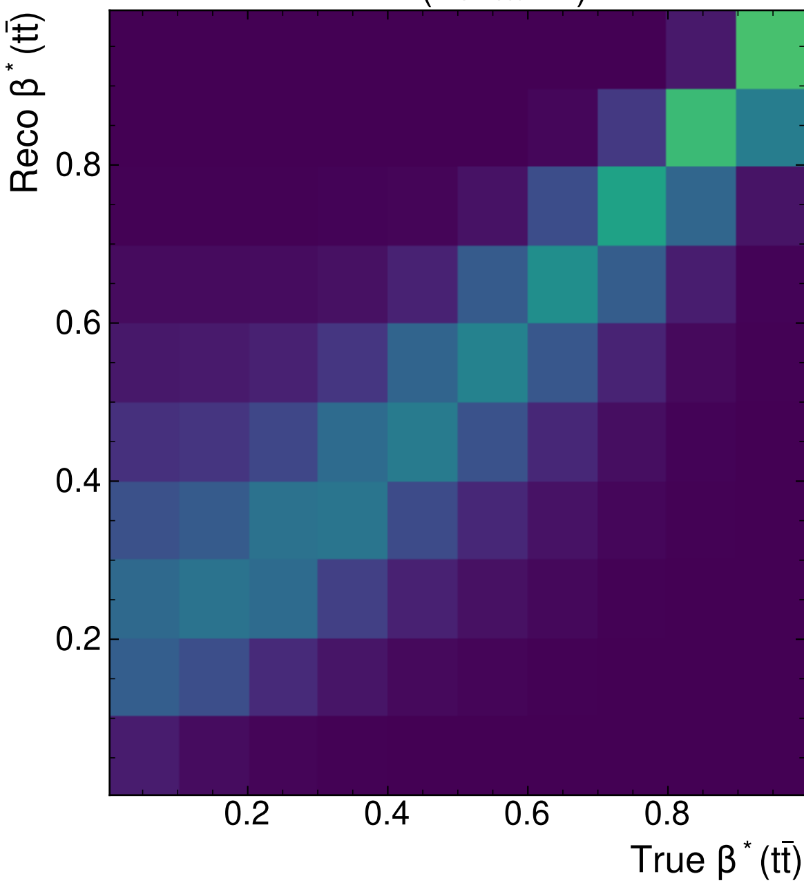
MMT (PtEtaPhi)
