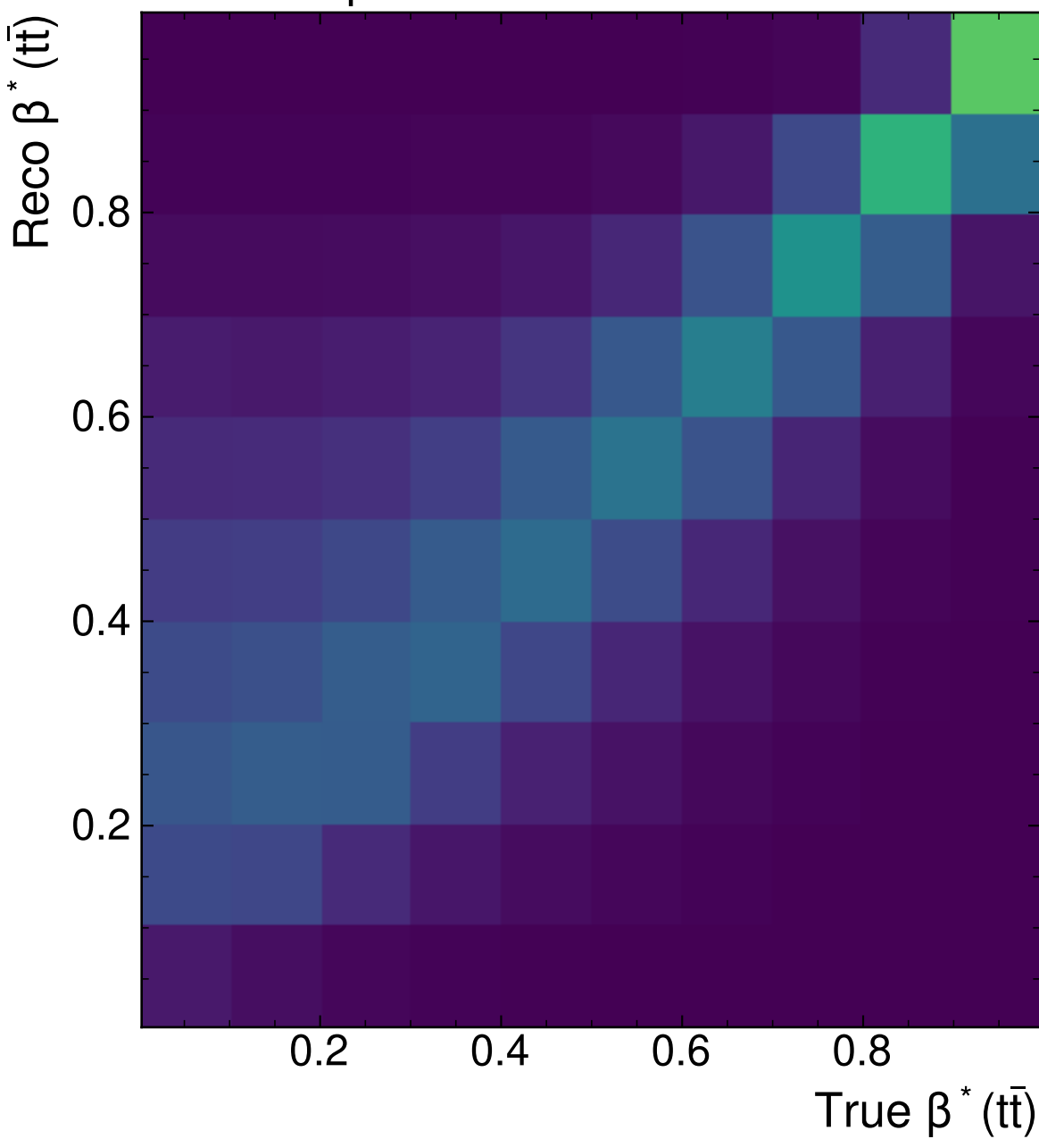
MMT (PtEtaPhi)
