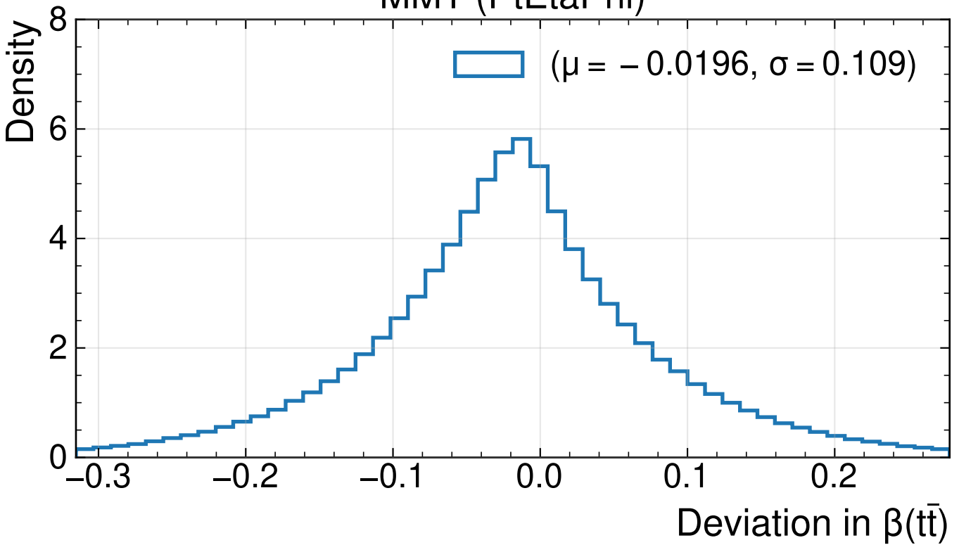
MMT (PtEtaPhi)
