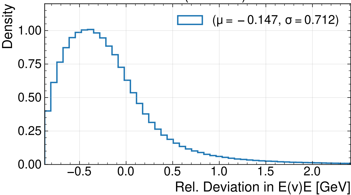
MMT (PtEtaPhi)
