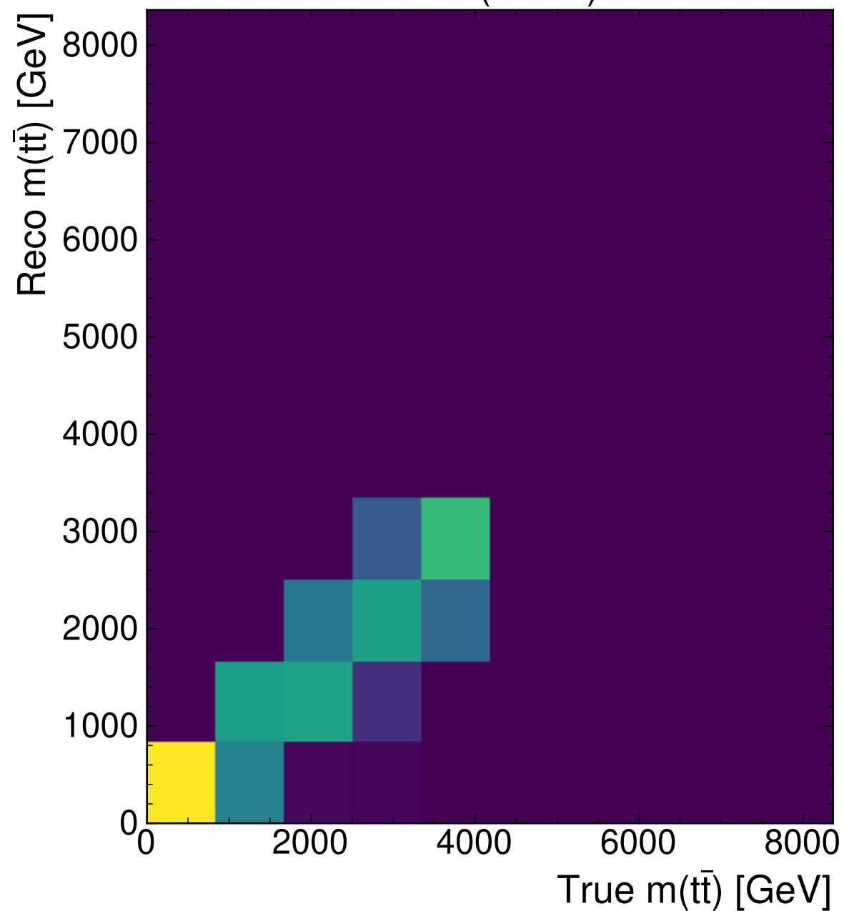
MMT (Mean)
