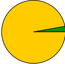
dilep_assigner_cr_emu
