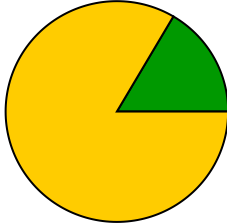
dilep_assigner_cr_mun
