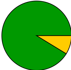
dilep_assigner_crZ
