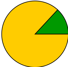
dilep_assigner_cr_ee
