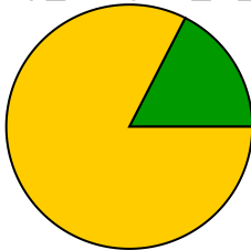
dilep_assigner_cr_mun
