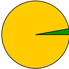
dilep_assigner_cr_emu
