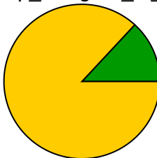
dilep_assigner_cr_ee
