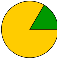
dilep_assigner_cr_mun
