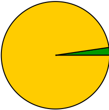
dilep_assigner_cr_emu
