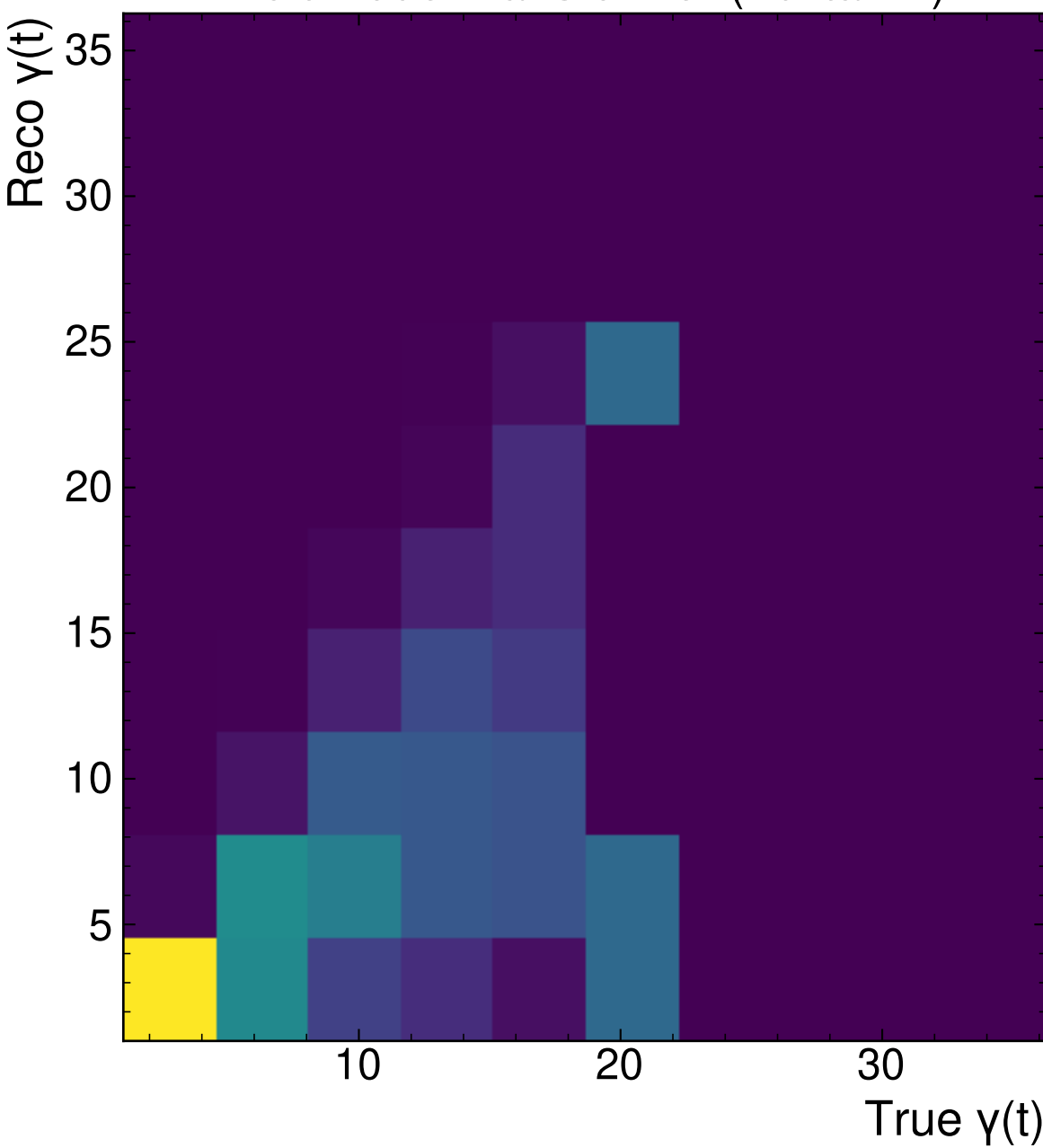
MultiModelTransformer (PtEtaPhi)
