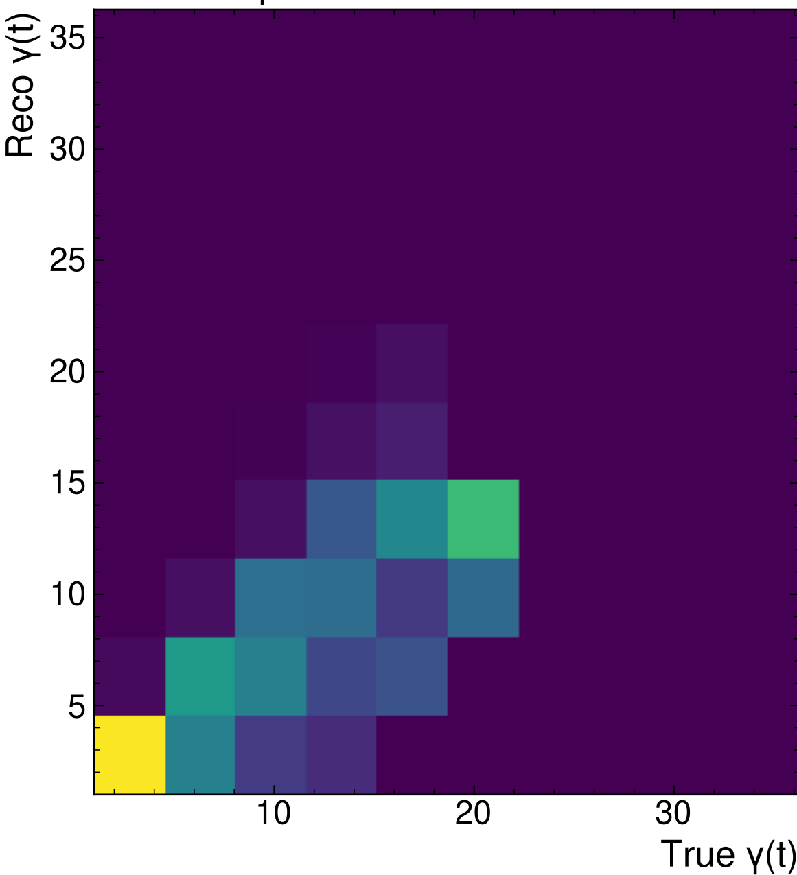
MultiModelTransformer (PtEtaPhi)
