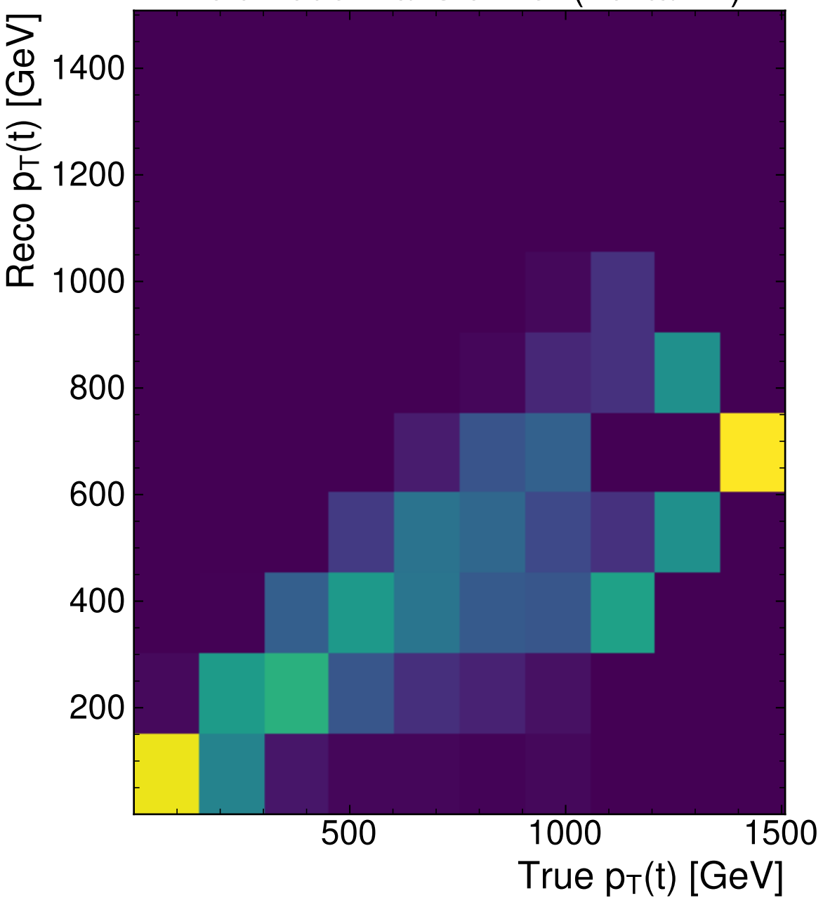
MultiModelTransformer (PtEtaPhi)
