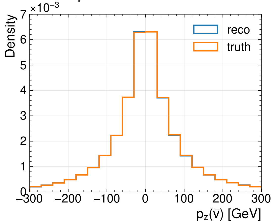
MultiModelTransformer (PtEtaPhi)
