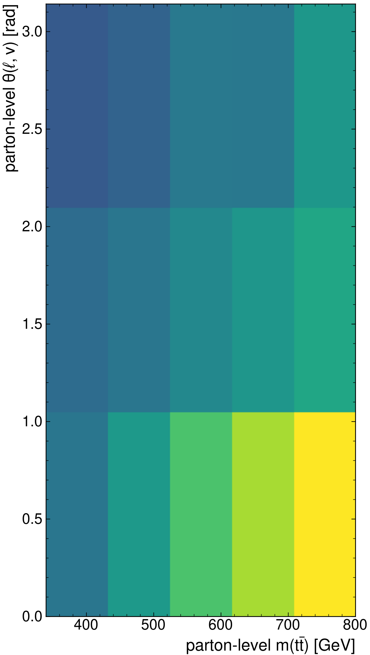
v 2 -Flows
