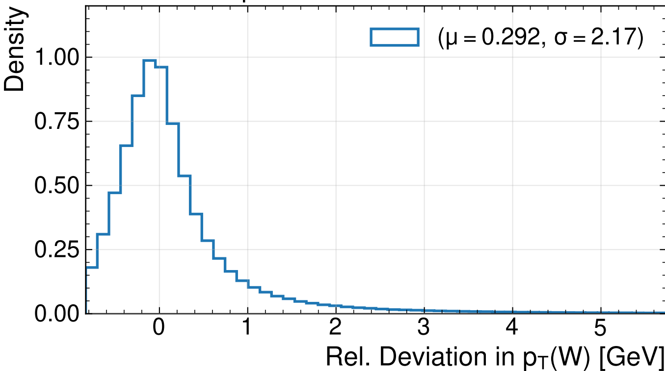
MMT (PtEtaPhi)
