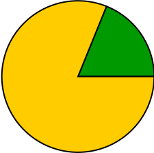
nu_flows_sr_mumu
