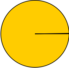
nu_flows_sr_emu
