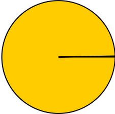
nu_flows_sr_emu
