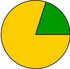
nu_flows_sr_mumu
