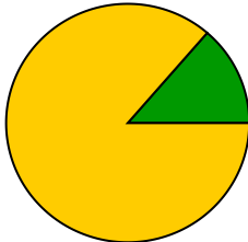
nu_weighter_cr_ee
