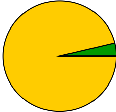
nu_weighter_cr_emu
