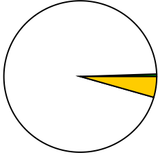
nu_flows_sr7
