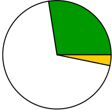
nu_flows_crZ
