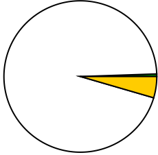
nu_flows_sr5
