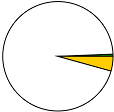
nu_flows_sr4
