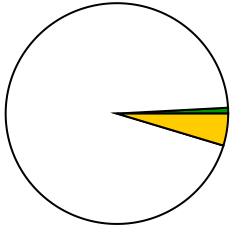
nu_flows_sr2
