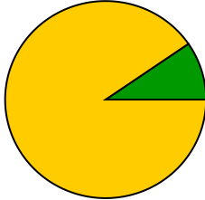
nu_flows_cr_ll
