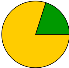
nu_flows_cr_mumu
