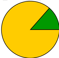
nu_flows_cr_ee
