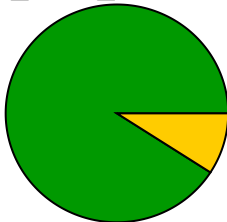
nu_flows_crZ
