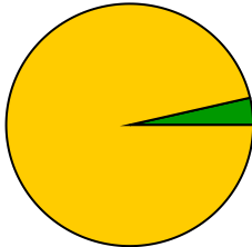
nu_flows_cr_emu
