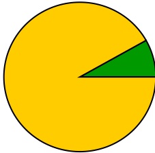
nu_flows_cr_ll
