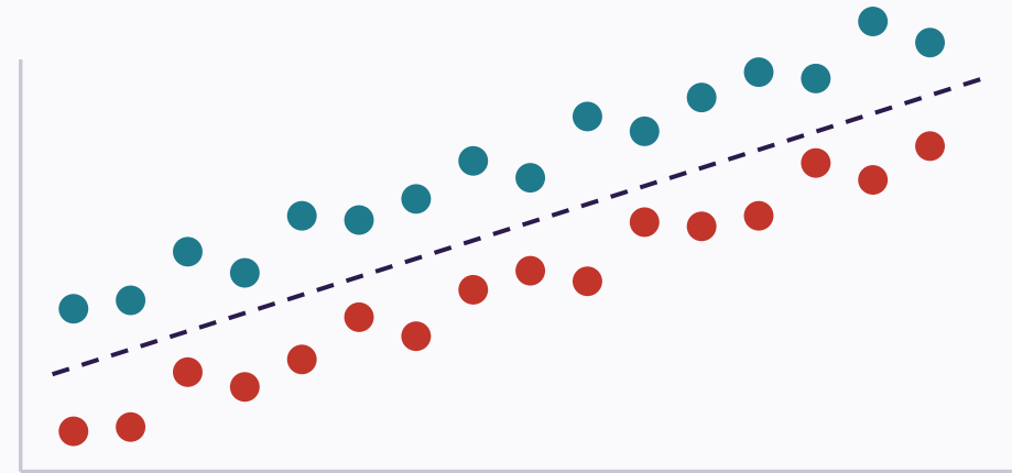
GENE-A × GENE-B
