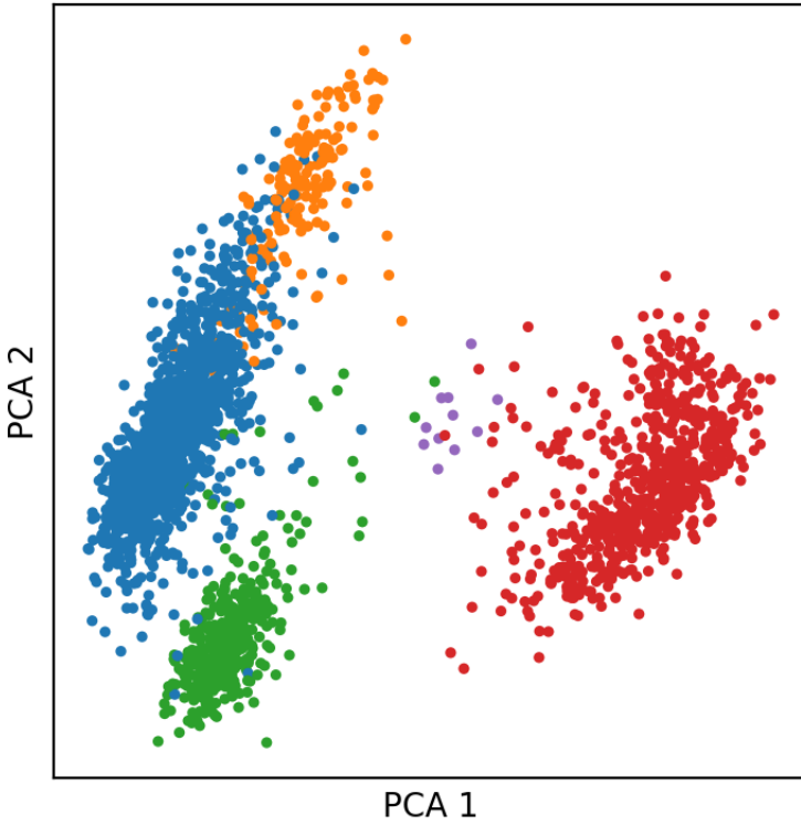
PCA
