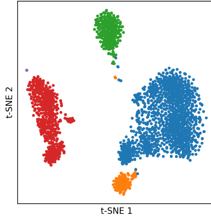
t-SNE
