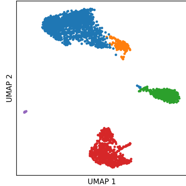
UMAP
