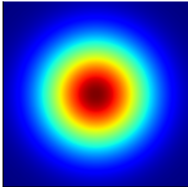
jet
