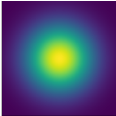
viridis
