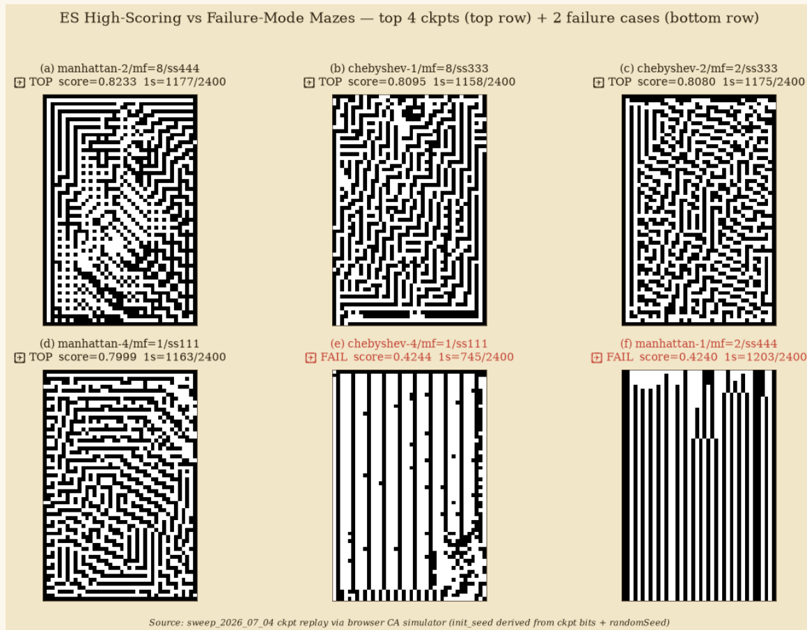
Figure 7 ES 跑出来的高分迷宫 (Top 1-3 + Top 5) 与重点特征失败模式 (Fail 1, Fail 2)。6 个 ckpt 在 300 步 CA 之后的 40 \times 60 终态。Top 1-3 的 maze_quality 均 \geq 0.81 , 4 个真迷宫共享 path-ratio \approx 0.48-0.49 (约半数通路半数墙), 即 maze attractor; Top 5 (manhattan-4 / mf=1) 是“均值降 / 峰值升”现象的体现: mf=1 的全局均值最低 (0.6984), 但 0.7999 的全场最高分就出现在 mf=1 上。Fail 1 (chebyshev-4 / mf=1) path-ratio 仅 0.31, 是“过稀疏”失败 ( 2^{103} 搜索空间 vs 10^5 预算, 大量“无梯度平台”让 CA 烧光活细胞); Fail 2 (manhattan-1 / mf=2) path-ratio 0.50 但“过连通”: 4 邻域只要求避让直接相邻的墙, 加上 mf=2 把墙推到最薄, CA 演化出几乎完全开放的网格, 缺乏走廊结构。
